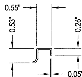
9 JAMB CLIP 1" LONG
